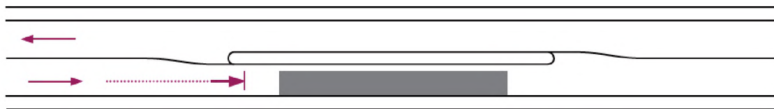
Obrázek 15 Autobusová (trolejbusová) zastávka na jízdním pruhu s fyzickým oddělením (zátku)- Typ IV
