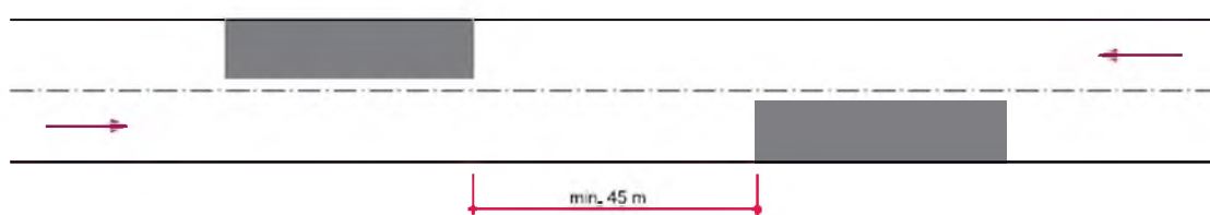
Obrázek 19 Umísťovanie zastávok c) - dvopruhovė komunikace, bez vyznačeného přechodu
