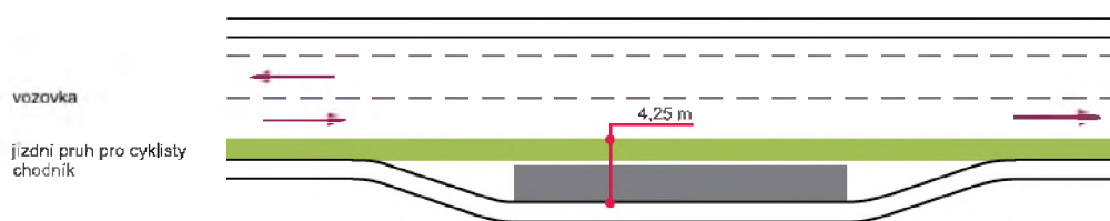
Obrázek 21 Provoz cyklistů v hlavním dopravním prostoru
