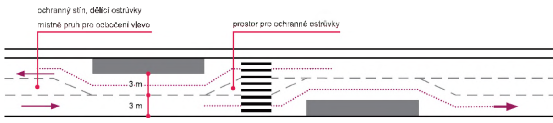
Obrázek 16 Autobusová (trolejbusová) zastávka na jízdním pásu s úpravou jízdnic pruhů - Typ II
